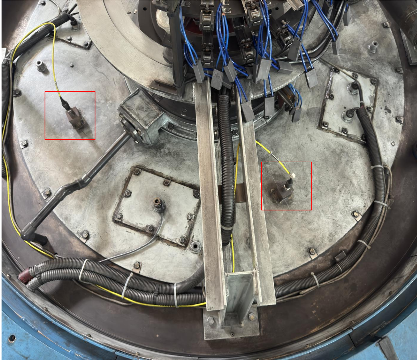
IV.3 - Các cảm biến rung lắp trực Rotor
