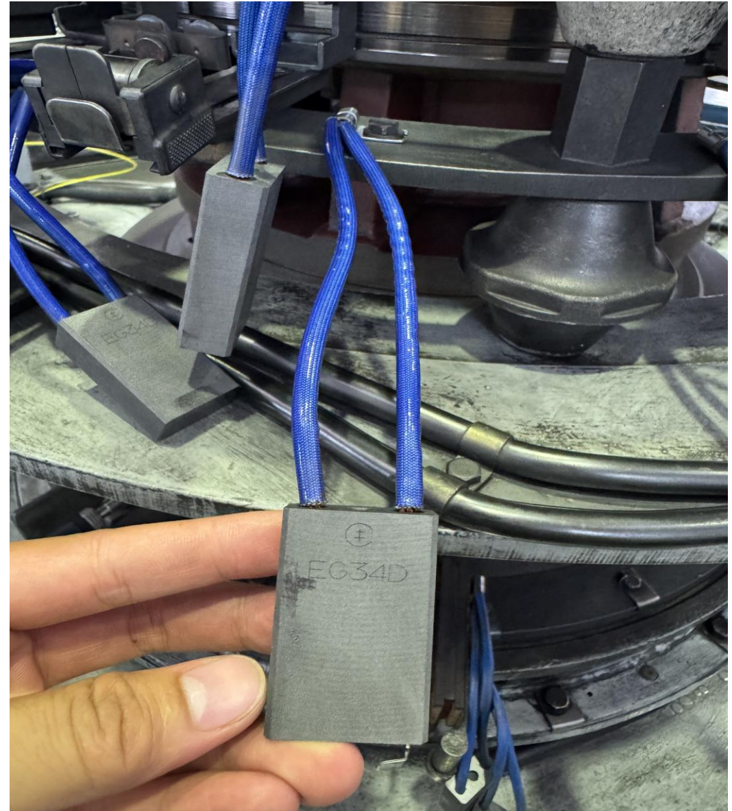
IV.2 Vành góp – chổi than
