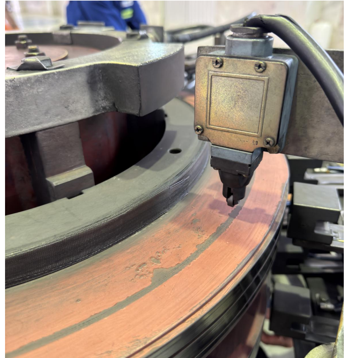
IV.5 Cảm biến vị trí TRÊN nâng trục Rotor
