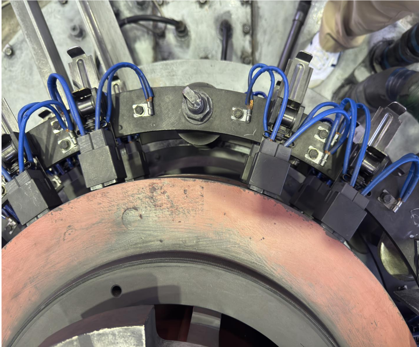
IV.2 Vành góp – chổi than
