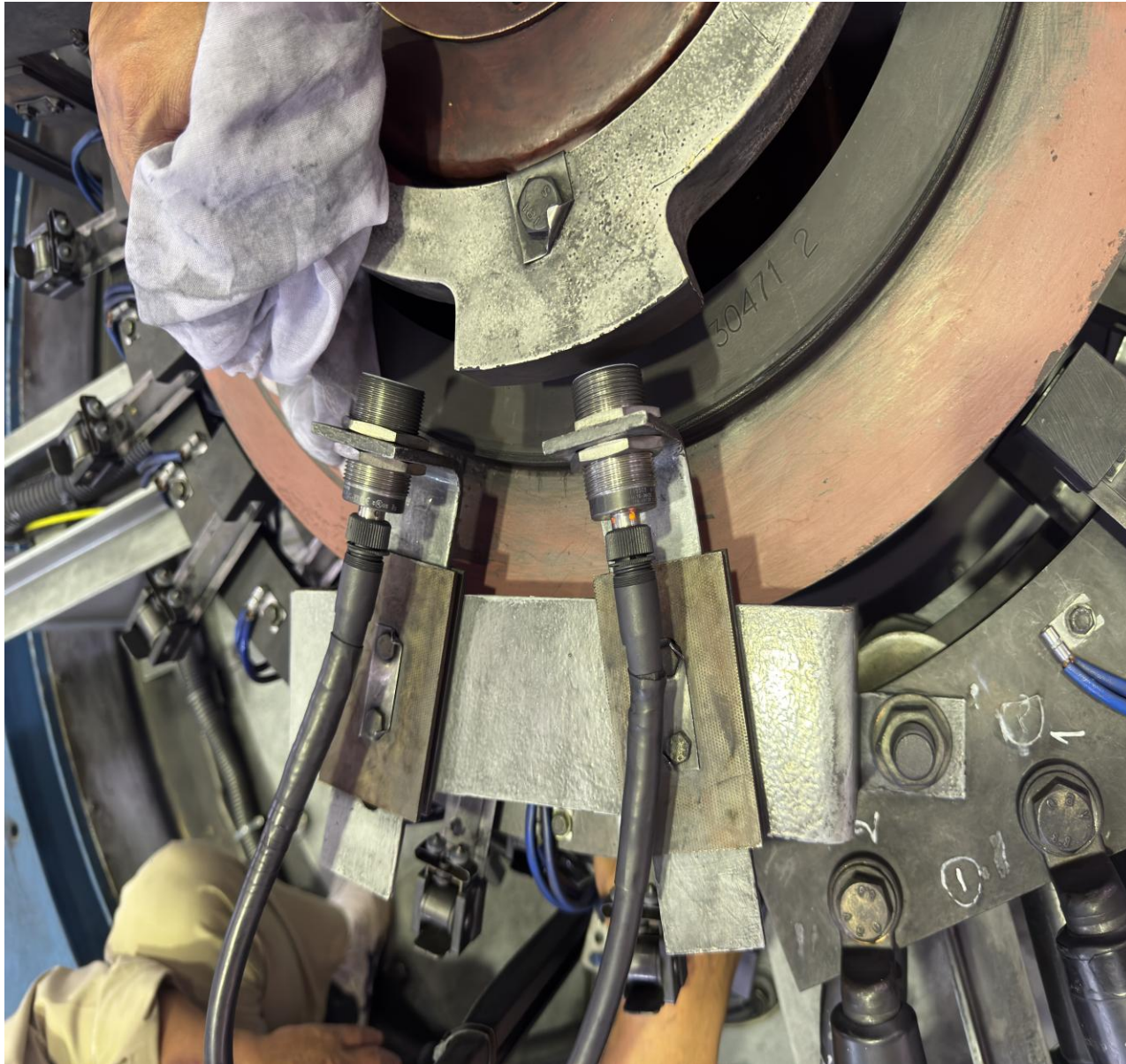
IV.4 - 02 cảm biến đo tốc độ quay Rotor
