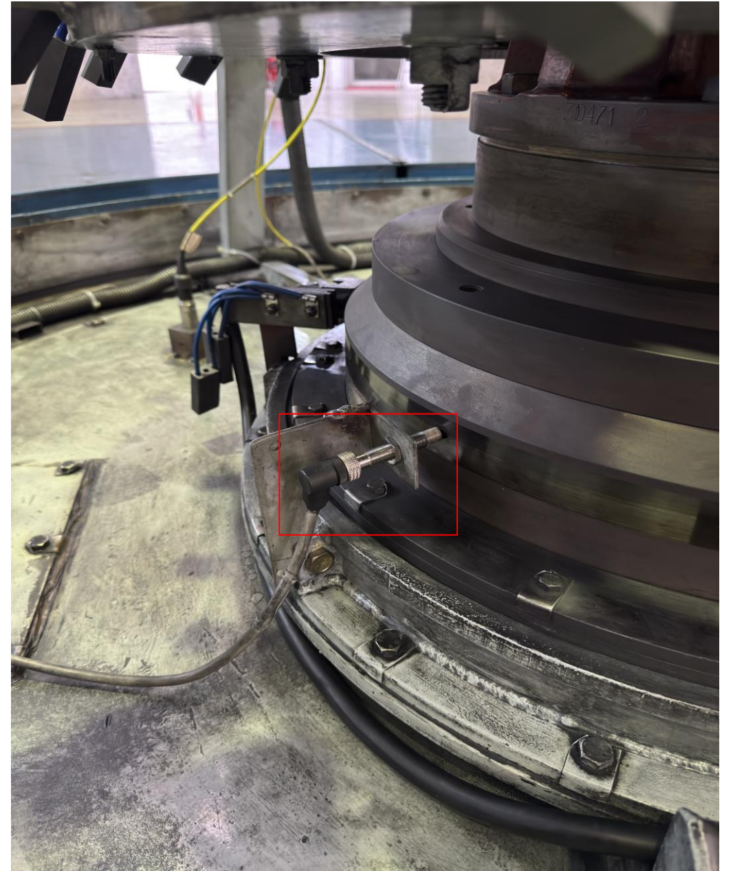
IV.3 - Các cảm biến rung lắp trực Rotor
